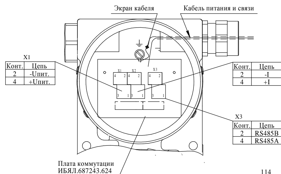
Рисунок платы коммутации газоанализаторов ДАК-СО2-131, ДАК-СН4-132, ДАК-ЭСН-133 с подходящими кабелями питания, связи
