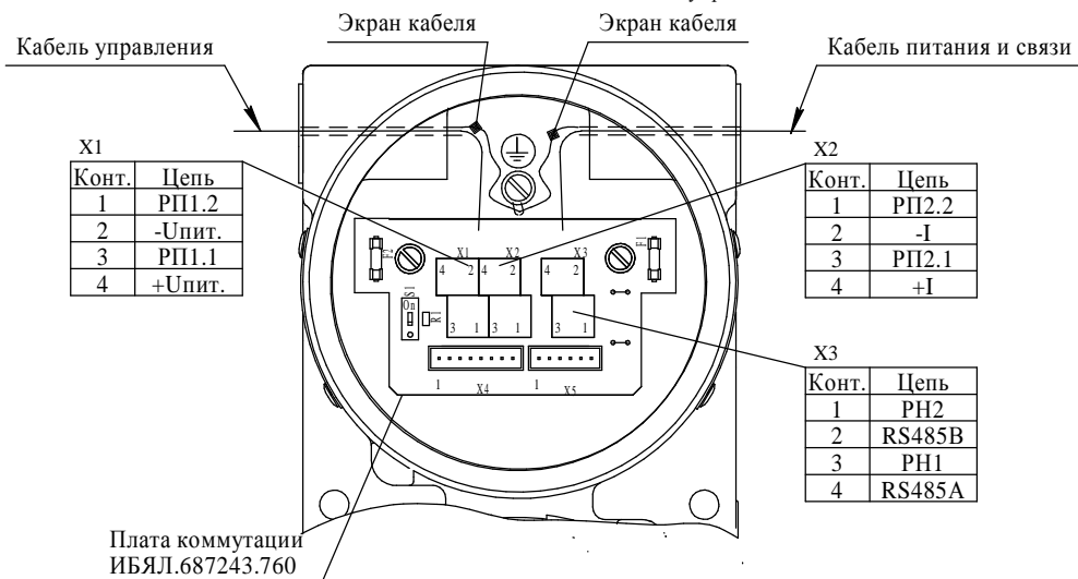
Рисунок платы коммутации газоанализаторов ДАК-СО2-126, ДАК-СН4-129, ДАК-СН4-137, ДАК-ЭСН-138, ДАК-ЭСН-139 с подходящими кабелями питания, связи, управления
