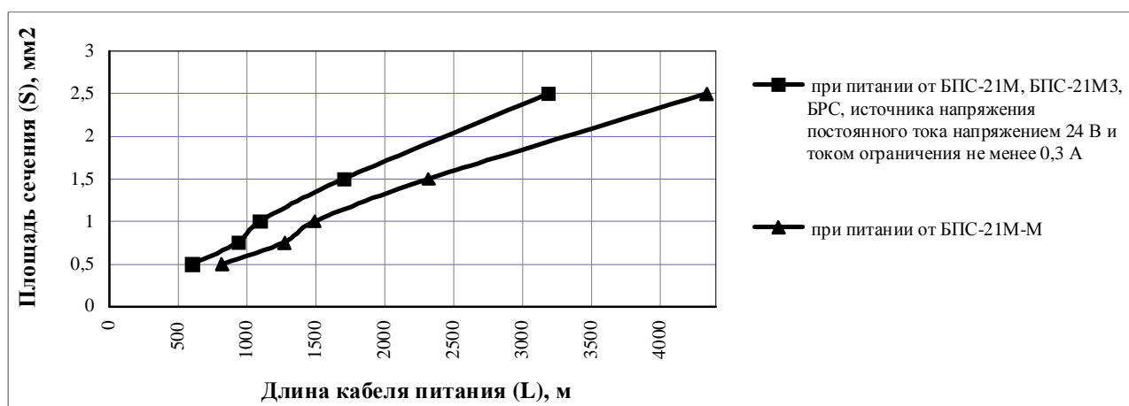
Рисунок И.2 – Зависимость площади сечения жилы кабеля питания от длины кабеля питания для газоанализаторов ДАК-СО 2 -126, ДАК-СН 4 -129, ДАК-СН 4 -137, ДАК-ΣСН-138, ДАК-ΣСН-139 при температуре окружающей воздуха от минус 40 °С до верхней границы диапазона рабочей (предельной) температуры (при отключенном подогреве)
