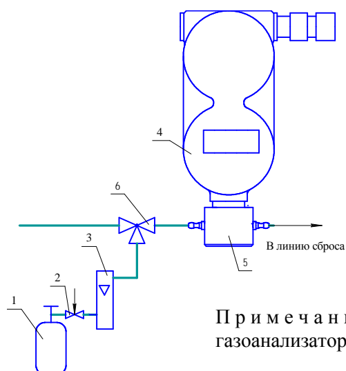
Рисунок 3.1 – Схема для проведения проверки (корректировки) нулевых показаний и чувствительности газоанализаторов
