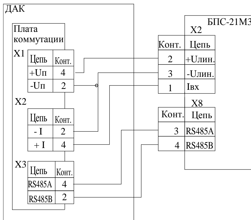
Рисунок Л.4 - Подключение газоанализаторов к БПС-21М3 ИБЯЛ.411111.047/-01/-02/-03/-04
