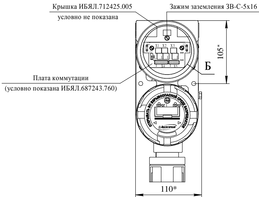
Рисунок платы коммутации газоанализаторов ДАК-СО2-126, ДАК-СН4-129, ДАК-СН4-137, ДАК-ЭСН-138, ДАК-ЭСН-139 с подходящими кабелями питания, связи, управления
