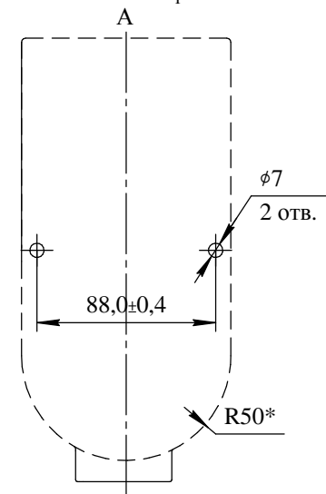
Рисунок платы коммутации газоанализаторов ДАК-СО2-131, ДАК-СН4-132, ДАК-ЭСН-133 с подходящими кабелями питания, связи
