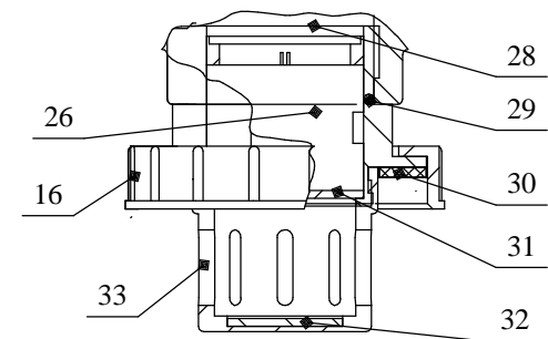
Рисунок 1.1 - Датчики-газоанализаторы ДАК-СО 2 -126, ДАК-СН 4 -129, ДАК-СО 2 -131, ДАК-СН 4 -132, ДАК-ΣСН-133, ДАК-СН 4 -137, ДАК-ΣСН-138, ДАК-ΣСН-139. Внешний вид
