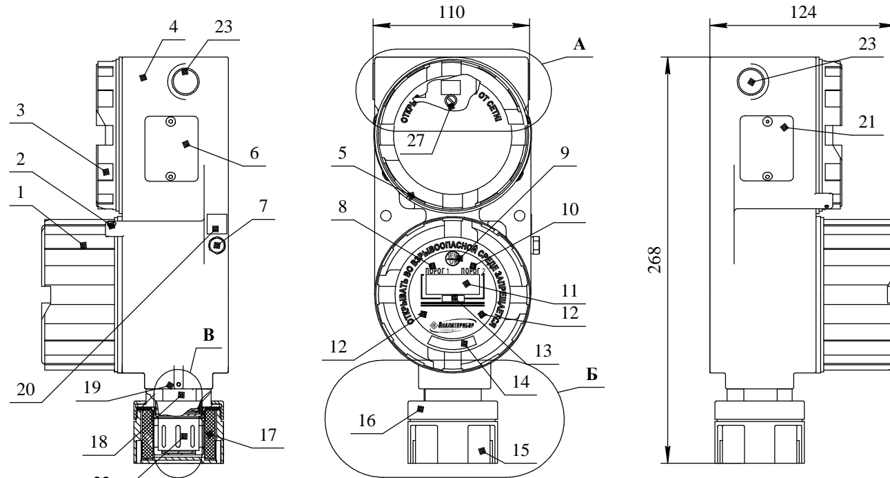
Рисунок внешнего вида газоанализаторов ДАК-СО 2 -131, ДАК-СН 4 -132, ДАК-ΣСН-133
