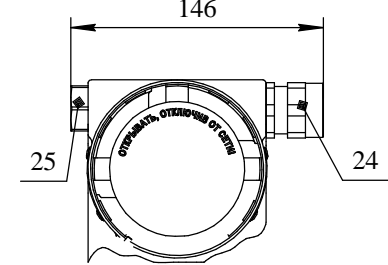
Рисунок внешнего вида газоанализаторов с установленным комплектом ИБЯЛ.305659.020
