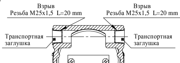
Рисунок Е.1 - Чертеж средств взрывозащиты газоанализаторов ДАК-СО 2 -126, ДАК-СН 4 -129, ДАК-СН 4 -137, ДАК-ΣСН-138, ДАК-ΣСН-139
