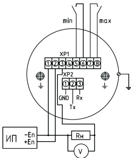
Рисунок В.12 – Прибор ДМ5002Вн-Г
