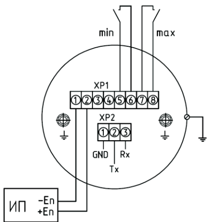
Рисунок В.11 – Прибор ДМ5002Вн-В
