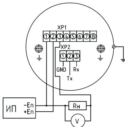
Рисунок В.10 – Прибор ДМ5002Вн-Б
