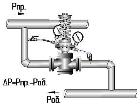
Рис.8 Включение регулятора УРД для поддержания перепада давления
