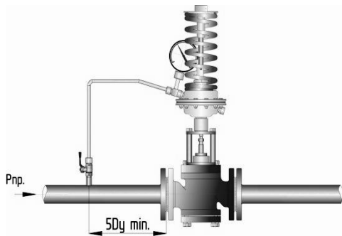
Рис.7 Включение регулятора УРД для поддержания давления
