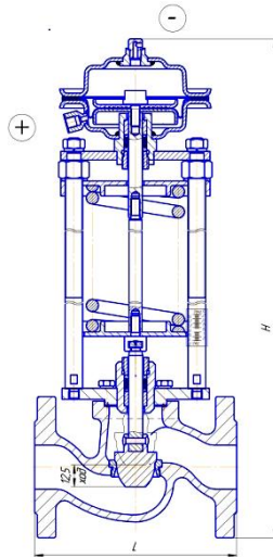
Рис.1 УРРД–НО-РД Ду25-80; УРРД – НЗ Ду 25-80 Рис.2 УРРД–НЗ-РПД Ду100-150
