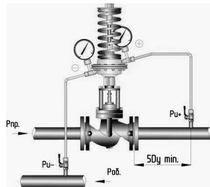
Рис.8 Включение регулятора УРД для поддержания перепада давления
