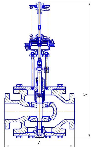
Рис.1 УРРД–НО-РД Ду25-80; УРРД – НЗ Ду 25-80 Рис.2 УРРД–НЗ-РПД Ду100-150
