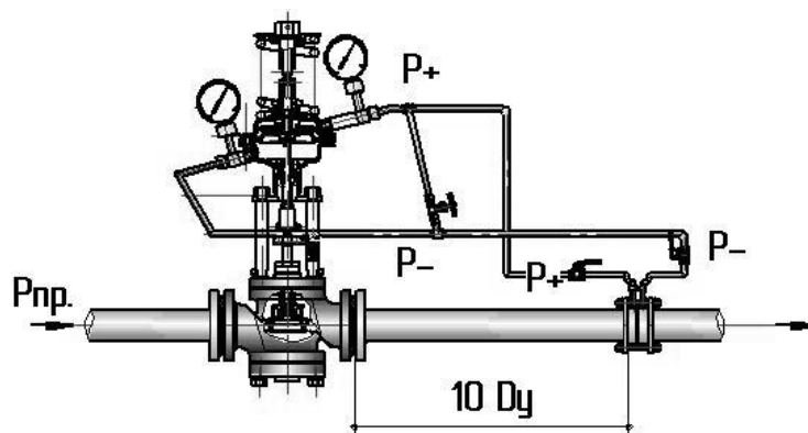
Рис.9 Включение регулятора УРД для поддержания расхода P_{пр} – давление потока регулируемой среды в прямом трубопроводе P_{об} – давление потока регулируемой среды в обратном трубопроводе
