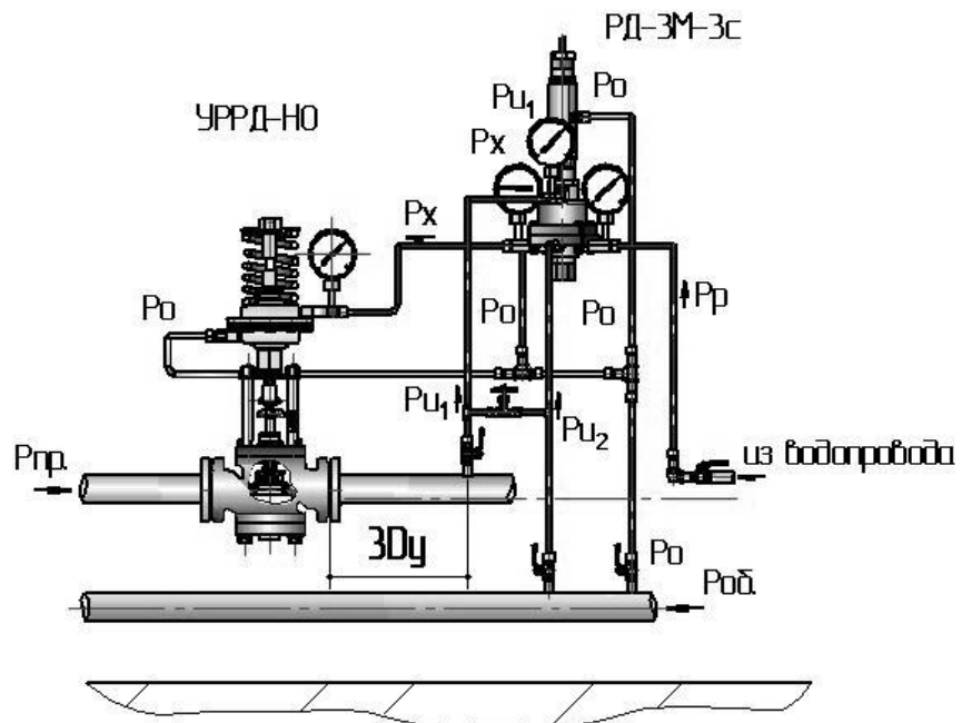
Рис.11 Бессливная схема регулирования давления «после себя».
