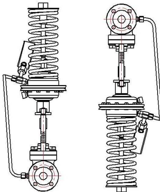
Рис.13 Рабочие положения регулятора УРРД
